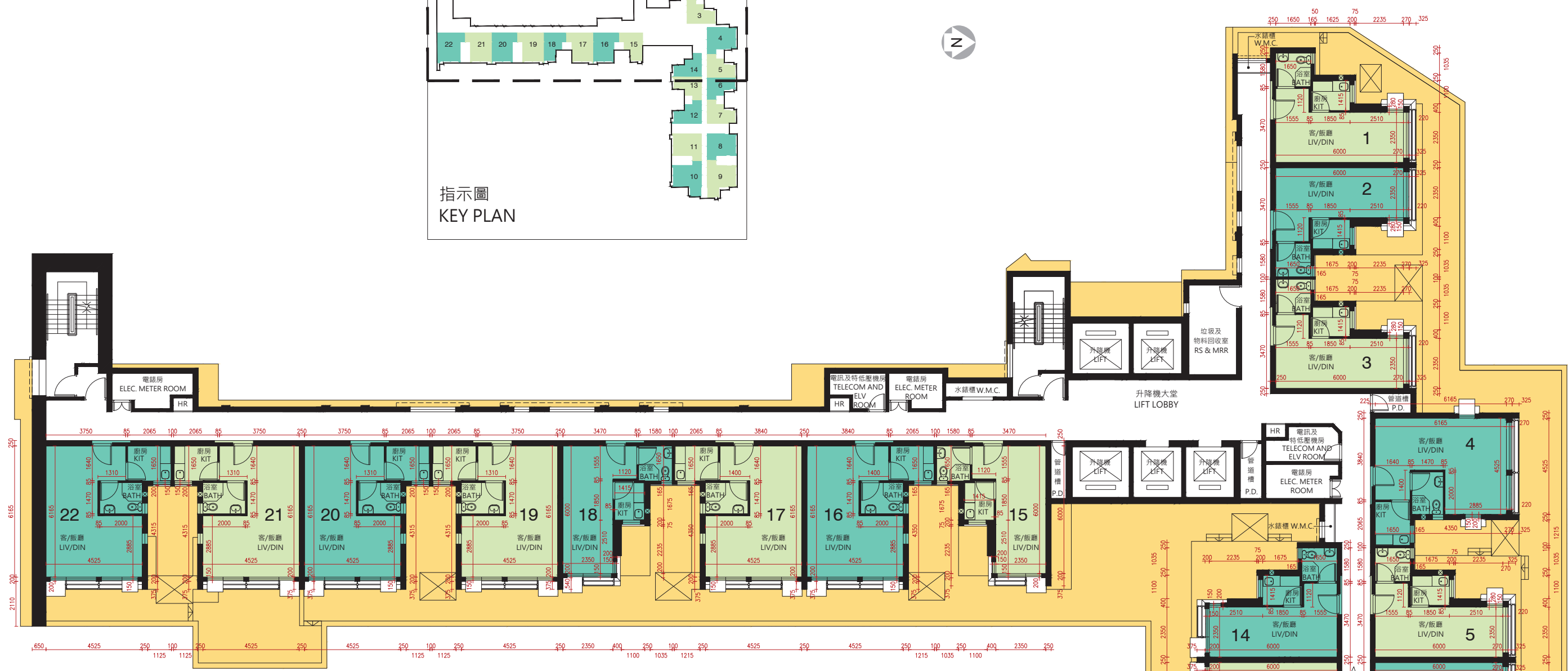
5樓平面圖 5/F Floor Plan
