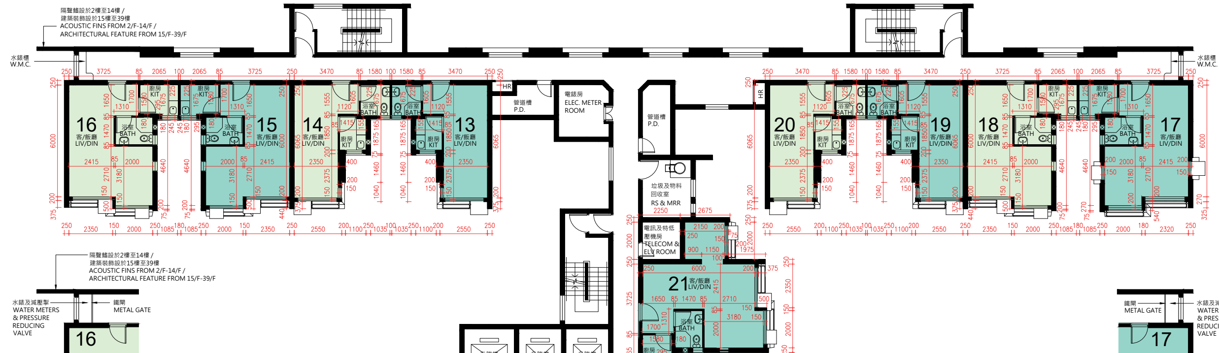
7樓、16樓及25樓部分平面圖 PART PLAN OF 7/F, 16/F & 25/F
