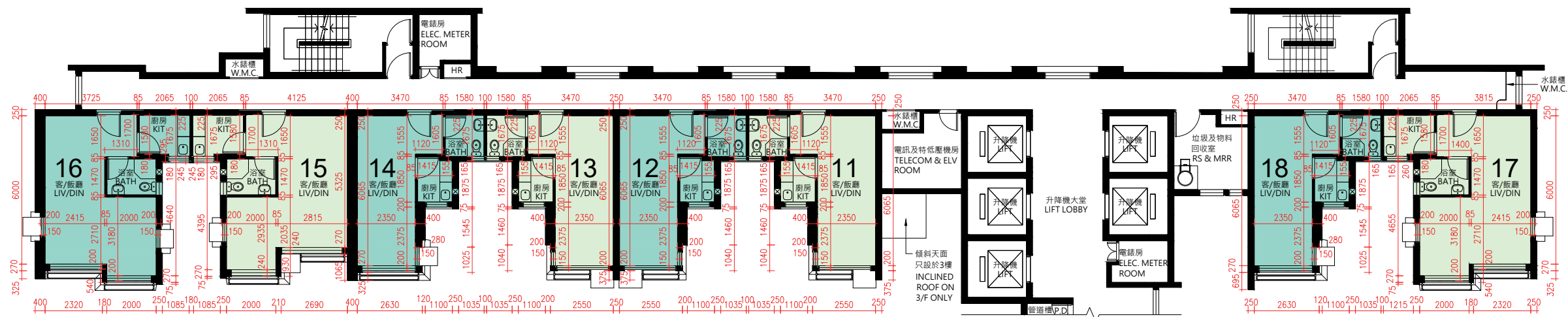
6樓、15樓及24樓部分平面圖 PART PLAN OF 6/F, 15/F & 24/F
