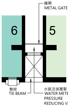
6樓、15樓及24樓部分平面圖 PART PLAN OF 6/F, 15/F & 24/F
