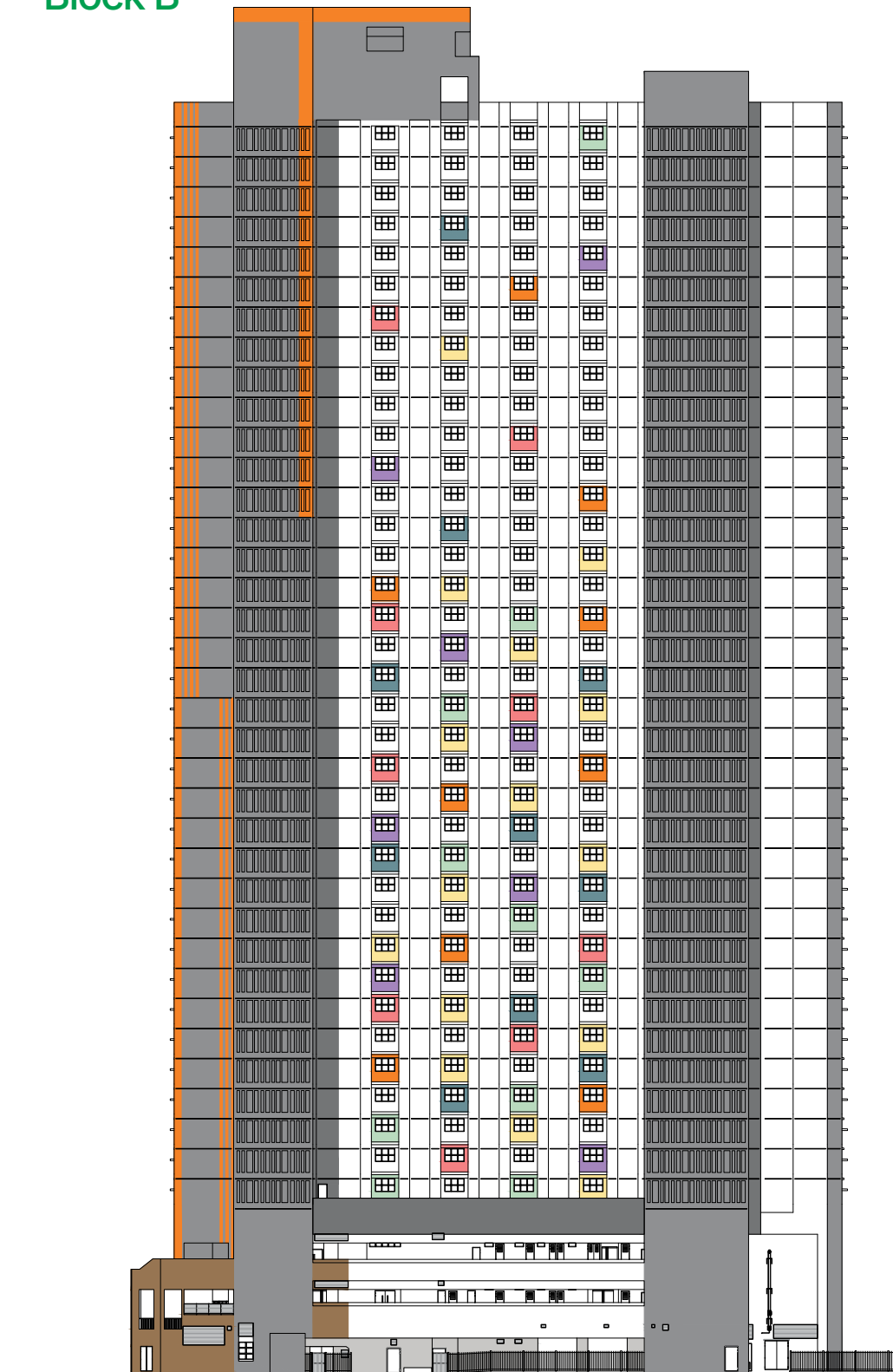
西北面立面圖 "7" North West Elevation Plan "7"
