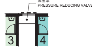
3樓、11樓及19樓部分平面圖 PART PLAN FOR 3/F, 11/F & 19/F
