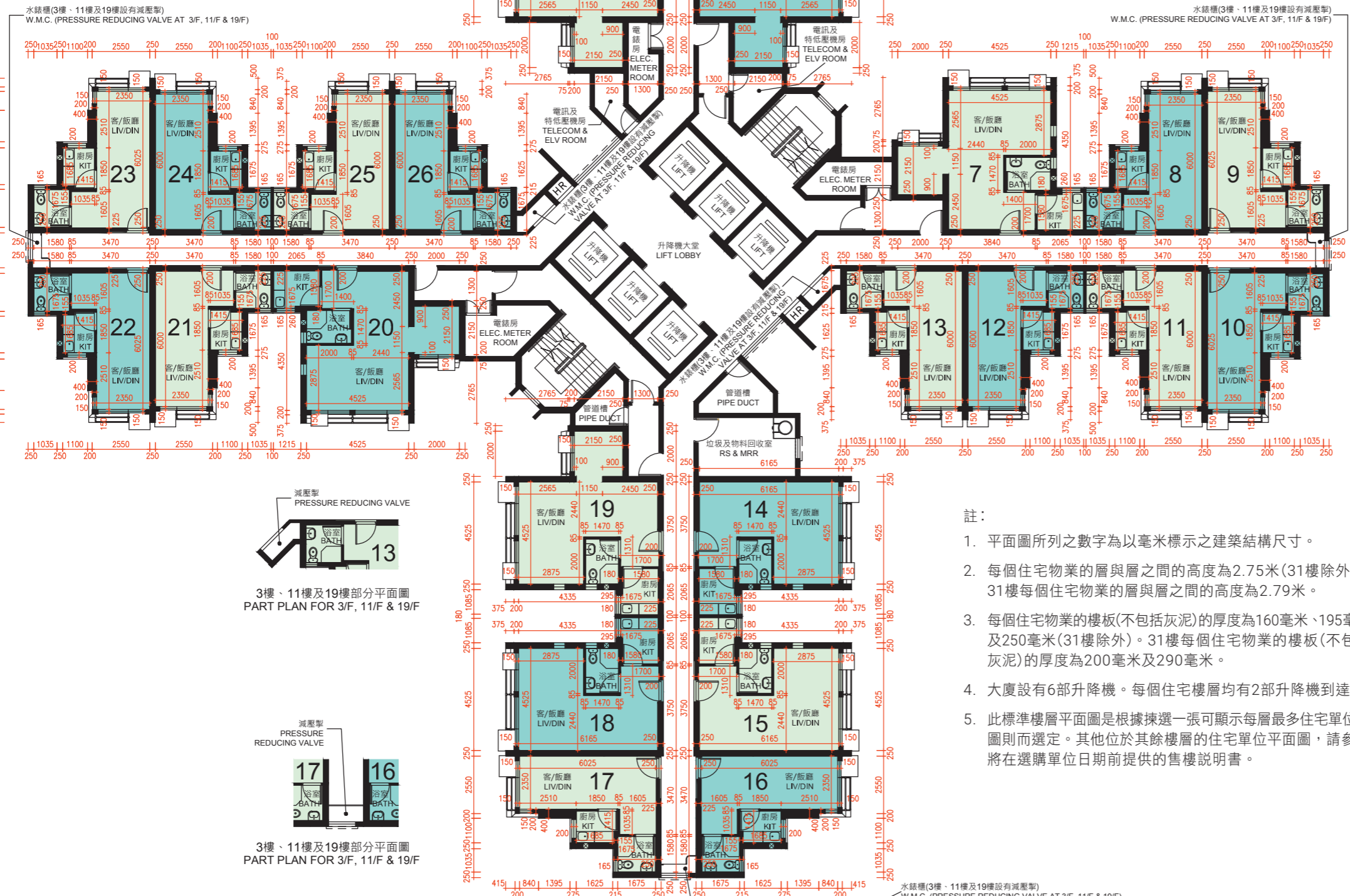
3樓、11樓及19樓部分平面圖 PART PLAN FOR 3/F, 11/F & 19/F
