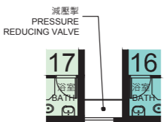
3樓、11樓及19樓部分平面圖 PART PLAN FOR 3/F, 11/F & 19/F
