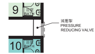
3樓、11樓及19樓部分平面圖 PART PLAN FOR 3/F, 11/F & 19/F
