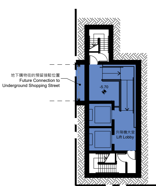
在香港主水平基準以下 5.70 米的部分平面圖 PART PLAN AT 5.70 METRES BELOW THE HONG KONG PRINCIPAL DATUM
