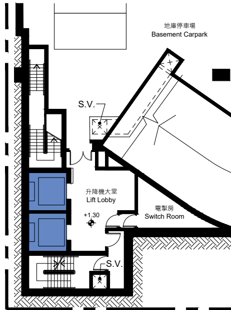
在香港主水平基準以上 1.30 米的部分平面圖(地庫停車場) PART PLAN AT 1.30 METRES ABOVE THE HONG KONG PRINCIPAL DATUM (BASEMENT CARPARK)
