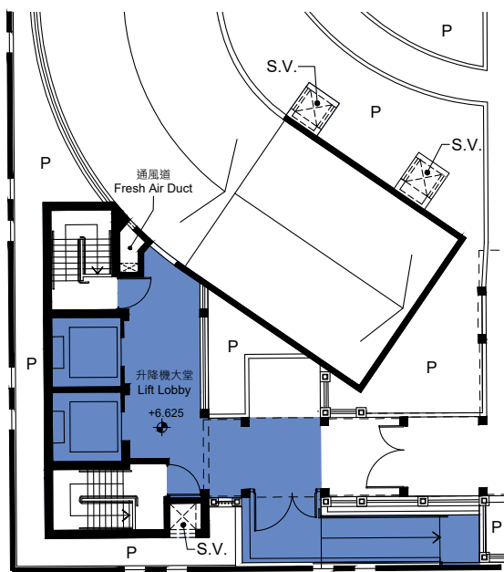
在香港主水平基準以上 6.625 米的部分平面圖(地下) PART PLAN AT 6.625 METRES ABOVE THE HONG KONG PRINCIPAL DATUM (GROUND FLOOR)
