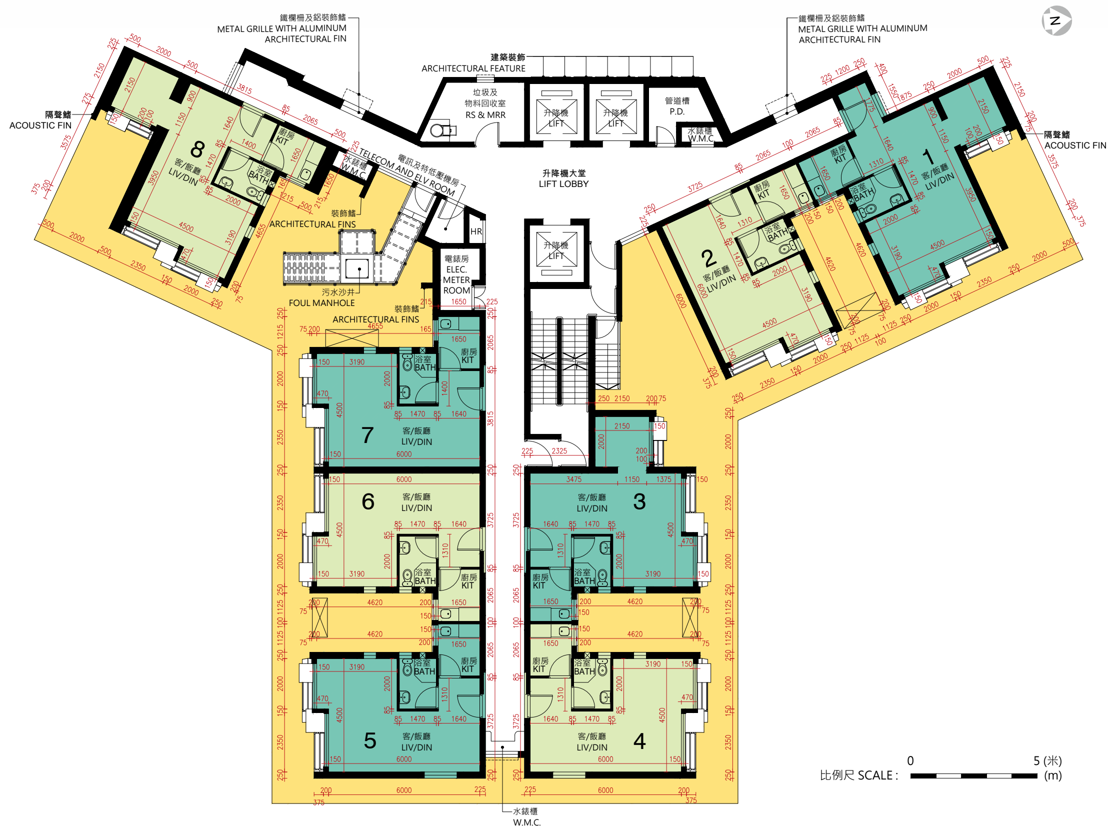
A座1樓平面圖 Block A 1/F Floor Plan
