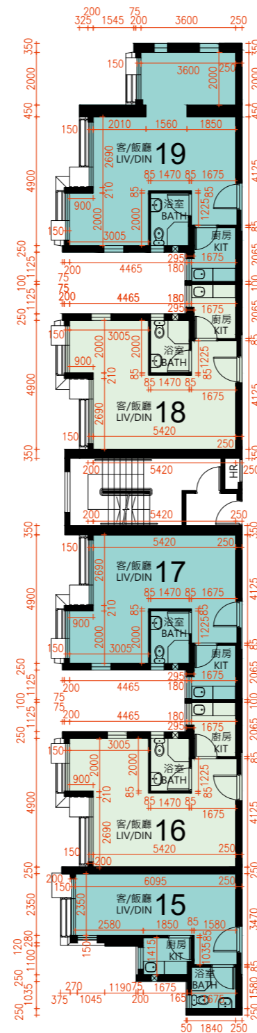
16樓至29樓部分平面圖 PART PLAN OF 16/F - 29/F
