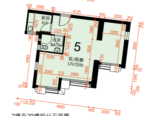
7樓至29樓部分平面圖 PART PLAN OF 7/F - 29/F
