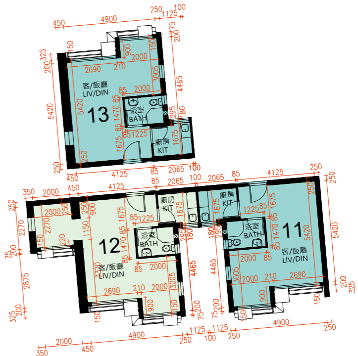
11樓至29樓部分平面圖 PART PLAN OF 11/F - 29/F
