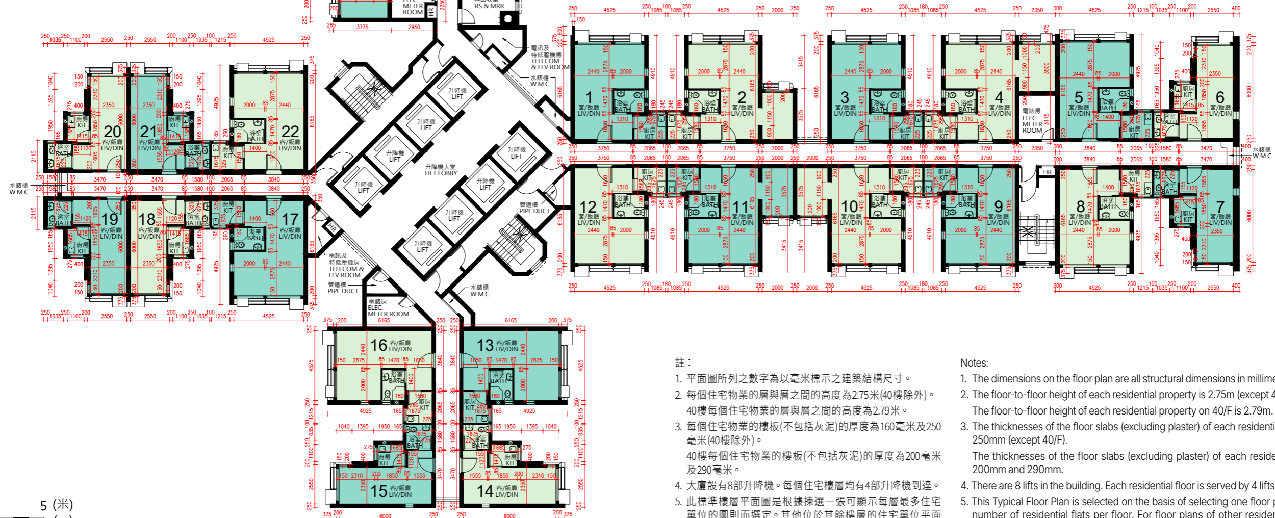
6樓、15樓及24樓部分平面圖 PART PLAN FOR 6/F, 15/F & 24/F
