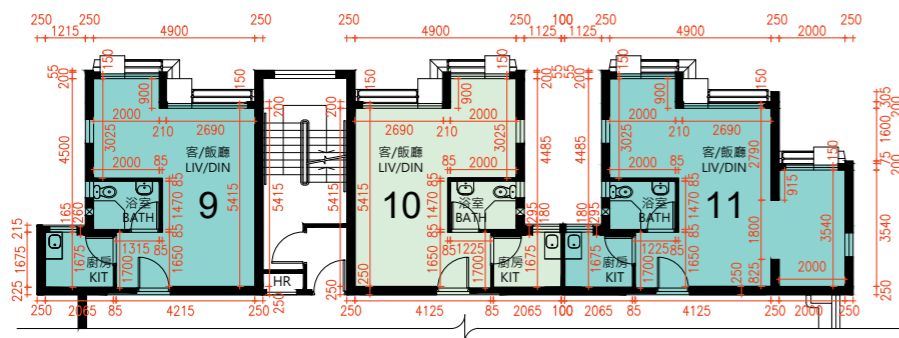
13樓至15樓部分平面圖 PART PLAN OF 13/F - 15/F
